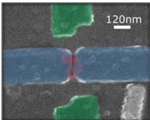
図2 素子の電子顕微鏡写真
