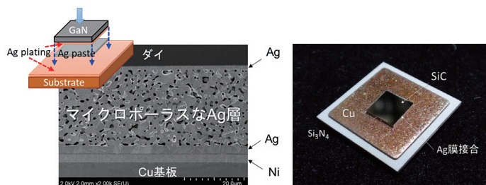
図 大気中、200℃、無加圧で完璧な接合が可能になる。 左) 接合界面、右) SiC を DBC へダイアタッチした例
