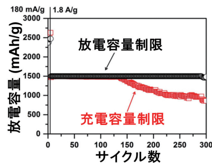
放電容量または充電容量を1500 mAh/gに制限したときのシリコンナノ粒子電極のサイクル特性
