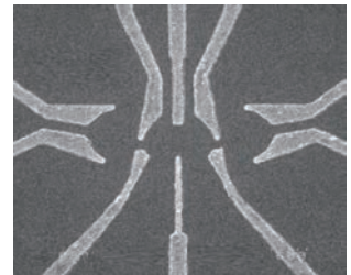
量子ドット
