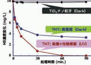
複合環境浄化機能：メチレンブルー色素除去特性
