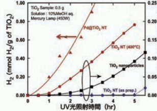
エネルギー創成機能：紫外線照射水分解水素発生性能
