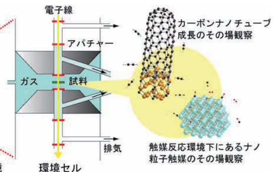
環境制御型透過電子顕微鏡
