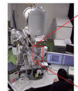
環境制御型透過電子顕微鏡
